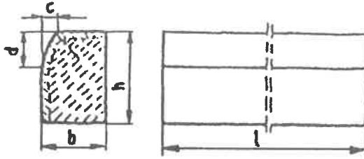
Rys. 1. Wymiarowanie krawężników
